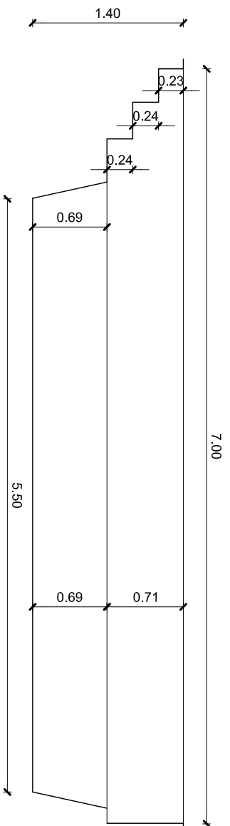
Sección
