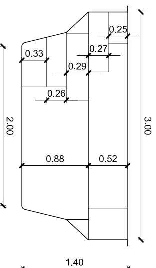
Alzado 2
