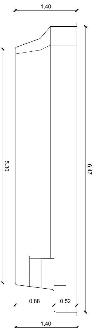
Seccion 1
